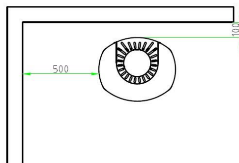
Mått till brännbar placering mot vägg
