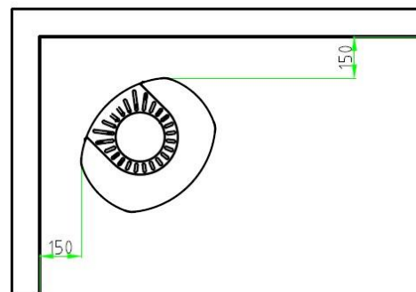
Mått till brännbar hörnplacering
